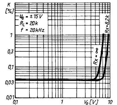
Bild 4: Klirrfaktor in Abhängigkeit von der Ausgangsspannung
