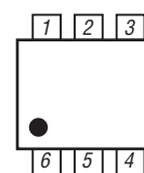
Bild 2: Pinbelegung (X65)
